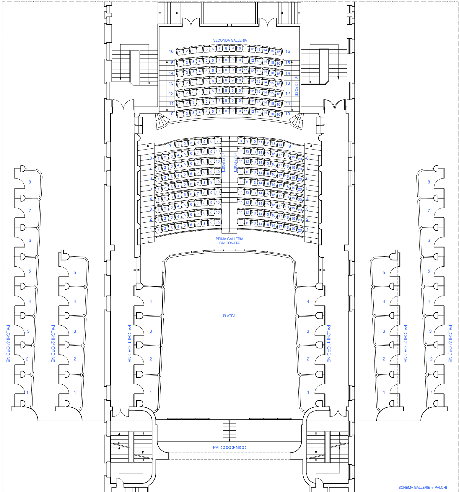
SCHEMA GALLERIE + PALCHI
